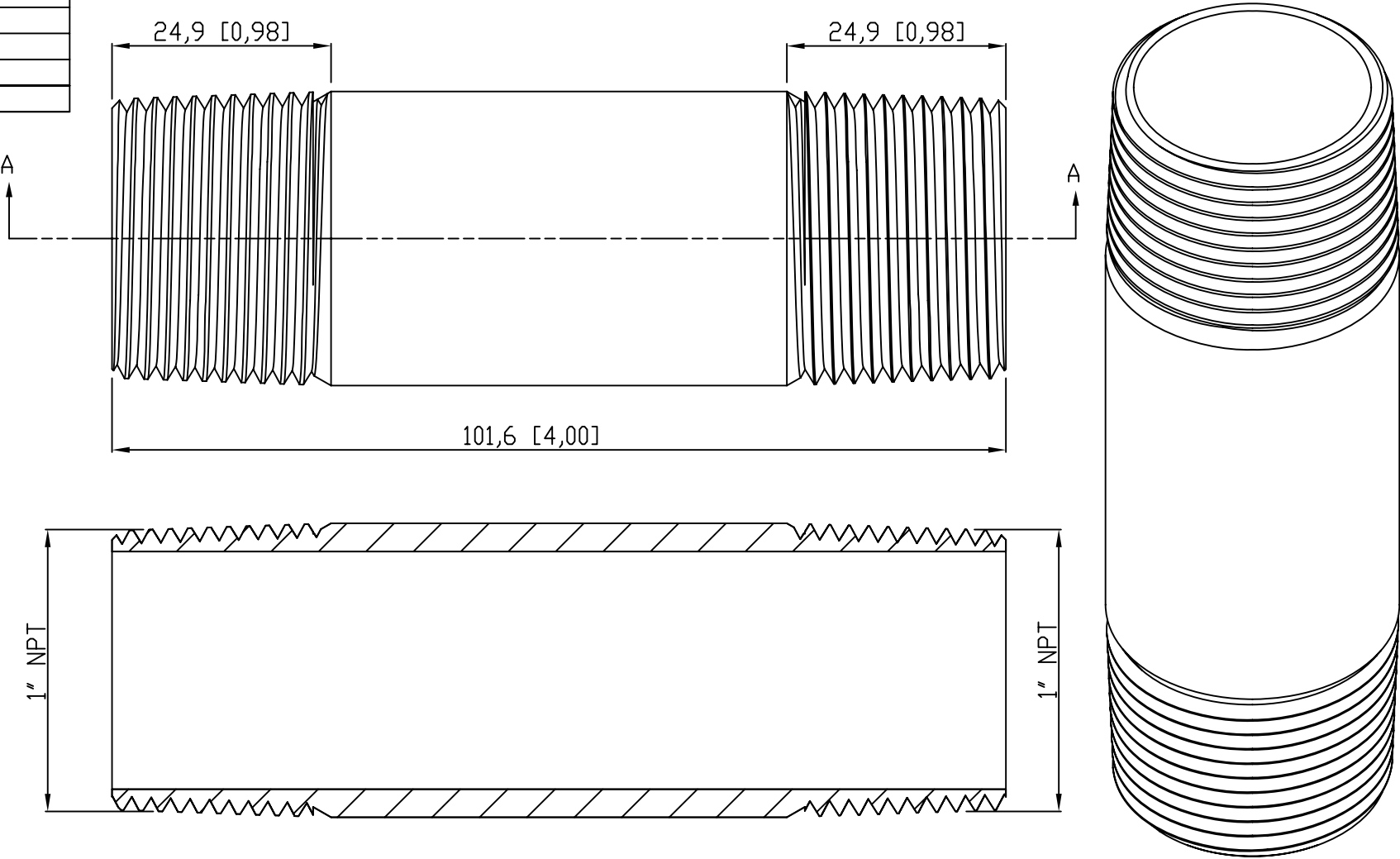
VIEW A-A
