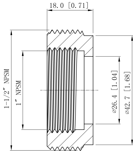
VIEW A-A
