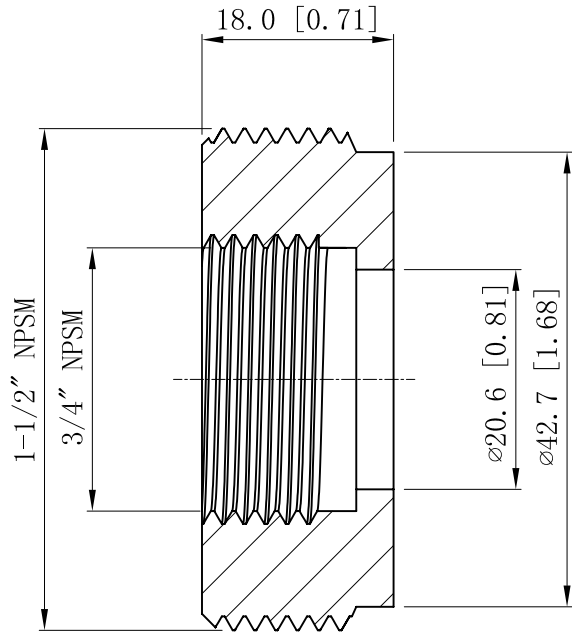
VIEW A-A
