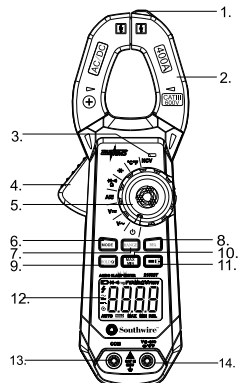
21550T Pince ampèremétrique Vue de face
