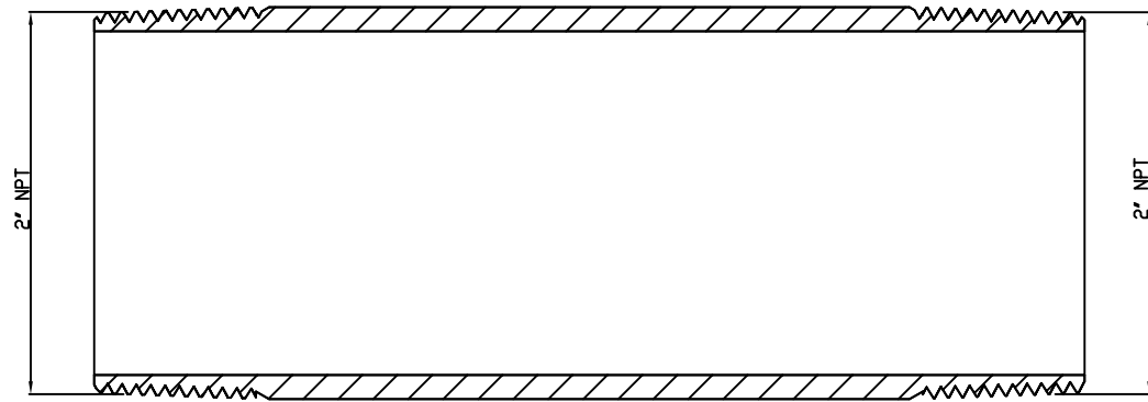
VIEW A-A
