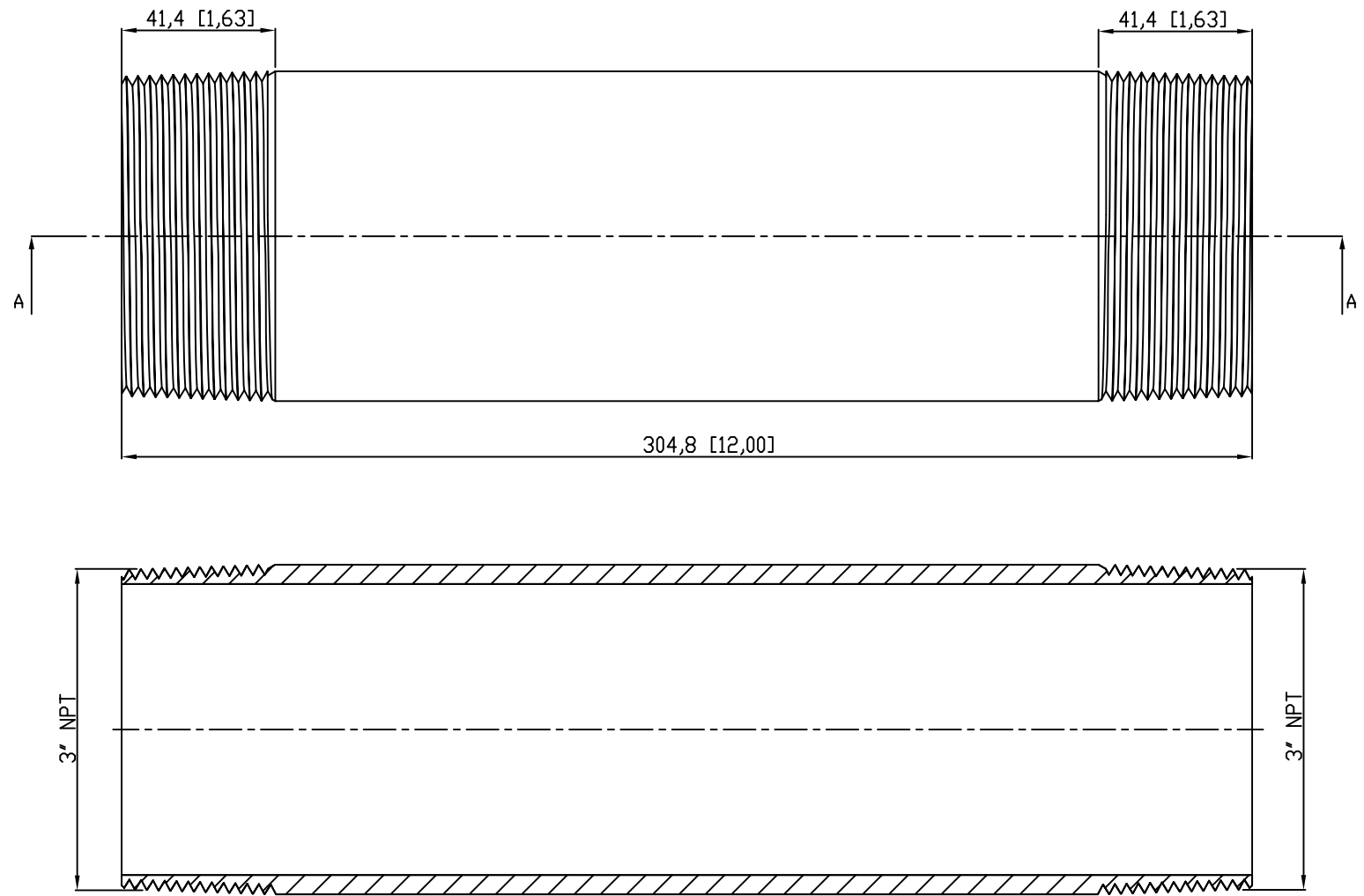
VIEW A-A
