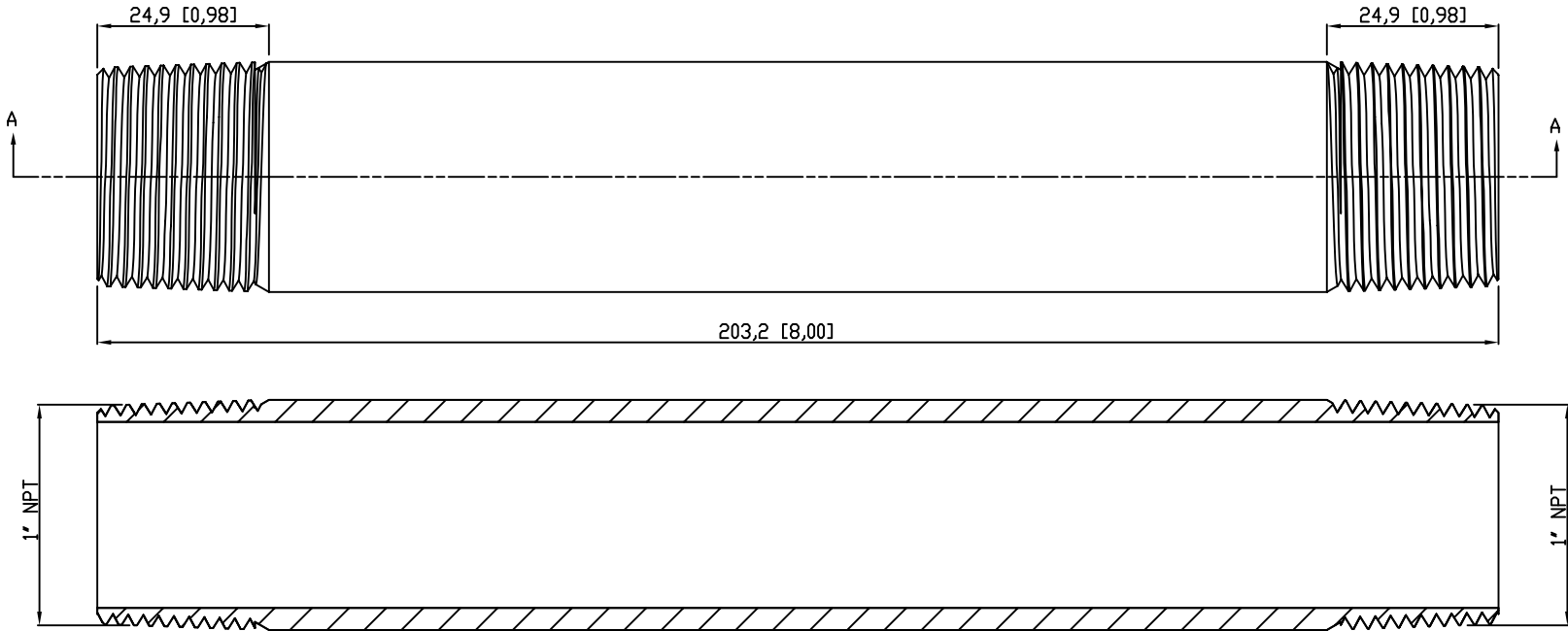
VIEW A-A
